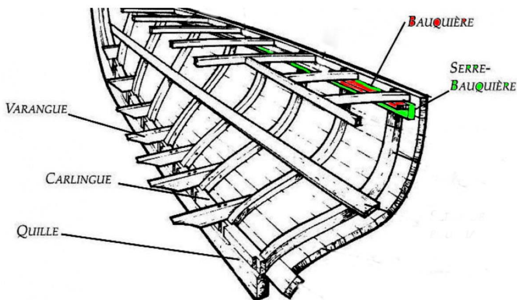
Coupe d'une coque
